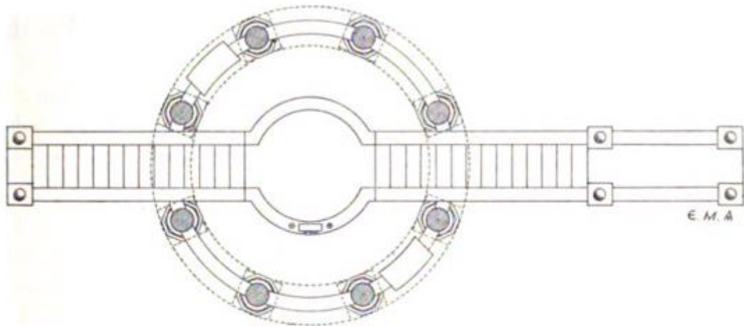
Σχ. 242. Ἀποκατάσταση τοῦ διαγράμματος τοῦ δευτέρου τῆς Ἁγίας Σοφίας Ἀμβωνος. Κλίμαξ=1½.
