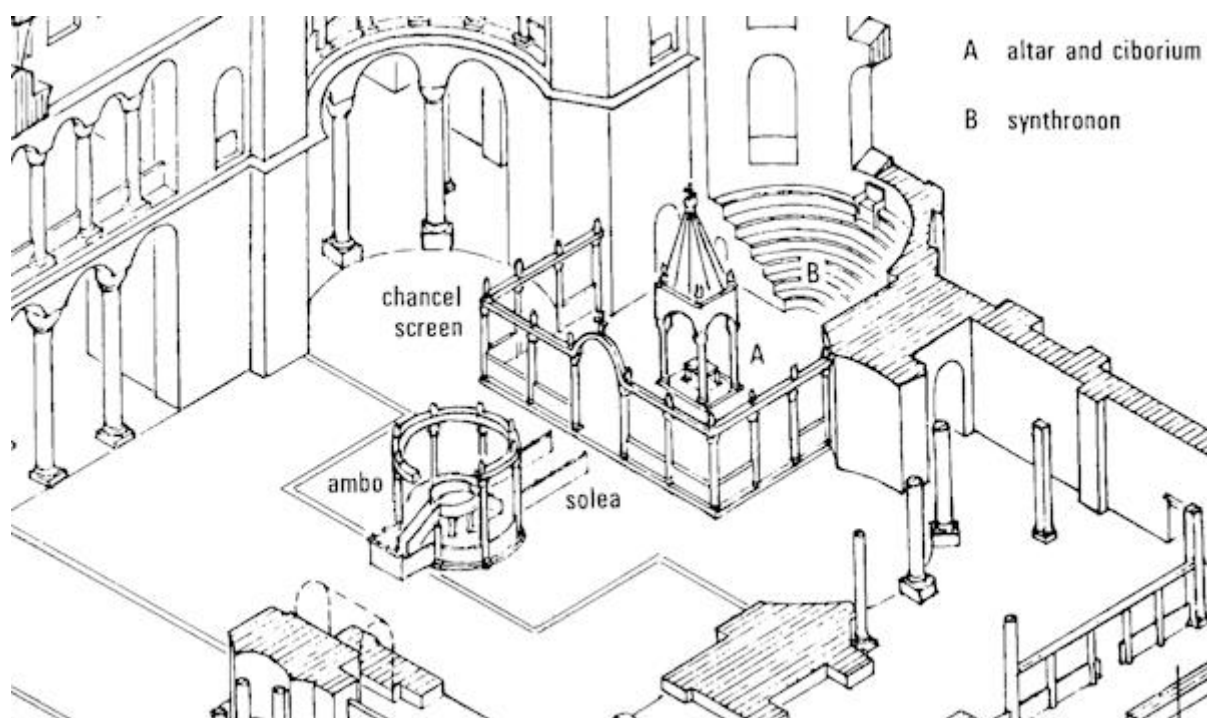
Είκ. 80-3. Ἑτέρα ἀπεικόνισις τῶν Κιγκλίδων / Τέμπλου, Ἀμβωνος, Ἱεροῦ τῆς Ἀγίας Σοφίας. 451
