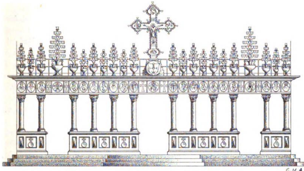
Σχ. 256. Ἀπόπειρα παραλήγοις ἀποκαταστάσεως τῶν Κιγκλίδων τοῦ Βήματος τῆς Ἁγίας Σοφίας. Κλίμαξ—188.
