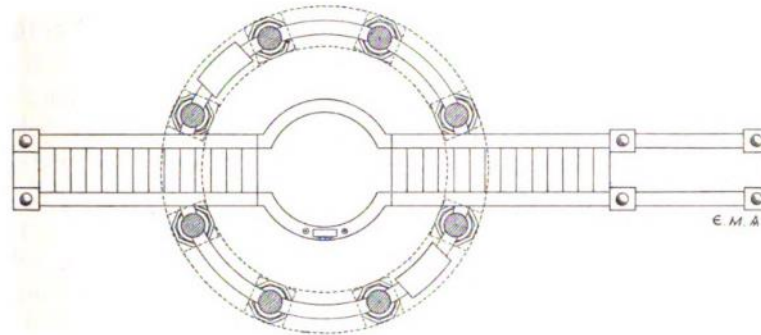
Σχ. 242. Ἀποκατάσταση τοῦ διαγράμματος τοῦ δευτέρου τῆς Ἁγίας Σοφίας Ἀμβωνος. Κλίμαξ=1½ε.
