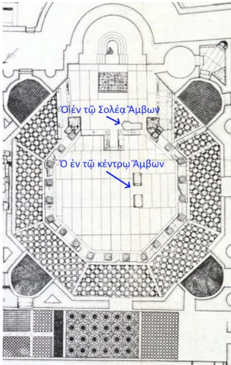
Εἰκ. 78-3. Ὀκταγωνικὴ Ἐκκλησίᾳ Φιλίππων, Στυλ. Πελεκανίδης, ΠΑΕ(1978), Μέρος ἐκ τοῦ Παρενθέτου Πίνακος Β'.
