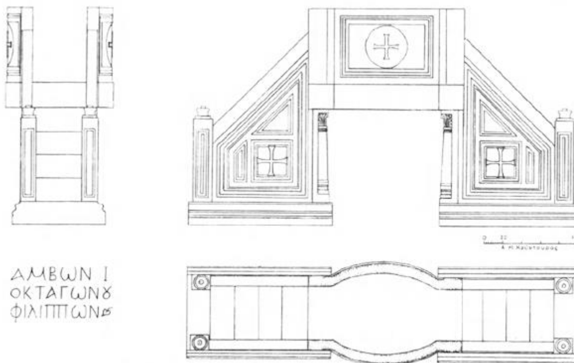
Εἰκ. 3. Ἀποκατάστασις τοῦ ἐν τῷ κέντρῳ τοῦ Ὁκταγώνου ἄμβωνος.
